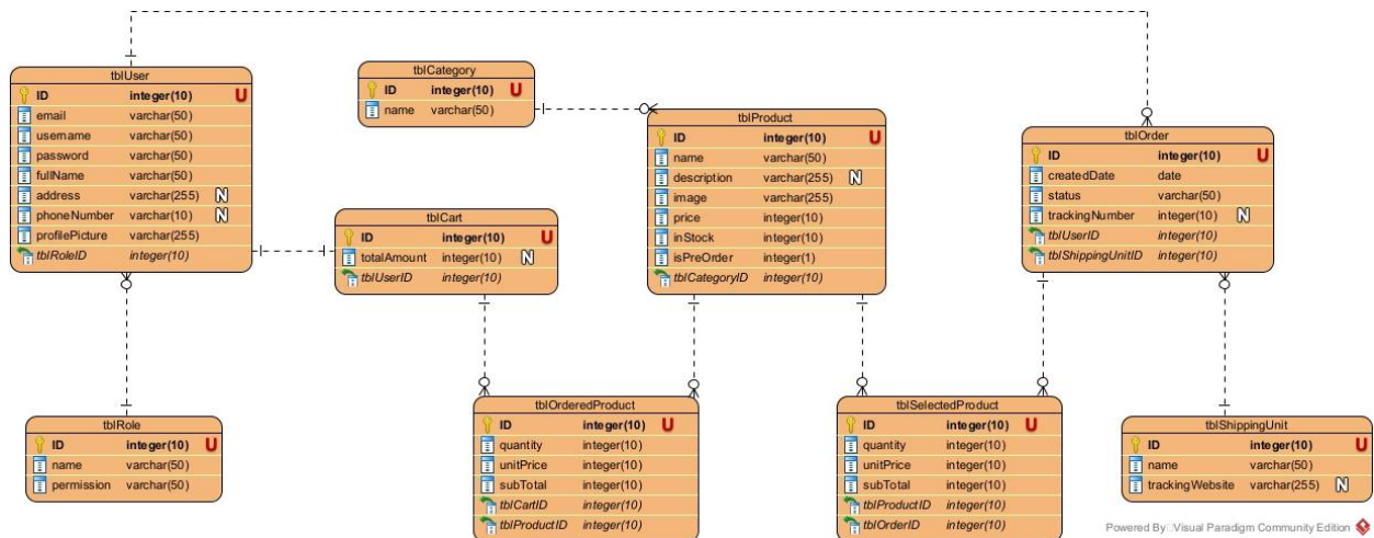
Hình 2.10. Thiết kế cơ sở dữ liệu của hệ thống
